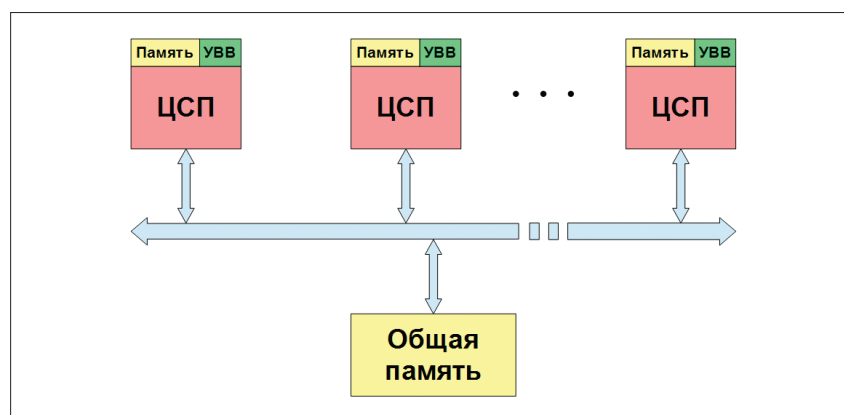
Рис. 2. Структурная схема SMP-системы на базе сигнального процессора 1967BH028
