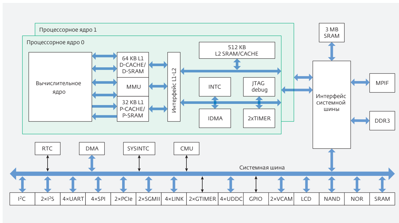
Рис.2. Структура процессора 1967BH058
