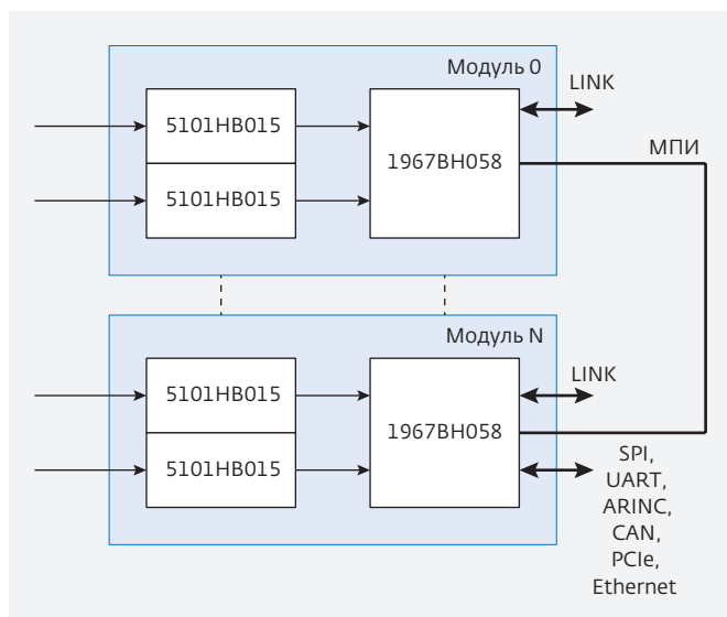
Рис.4. Многоканальная система обработки на процессорах 1967BH058
