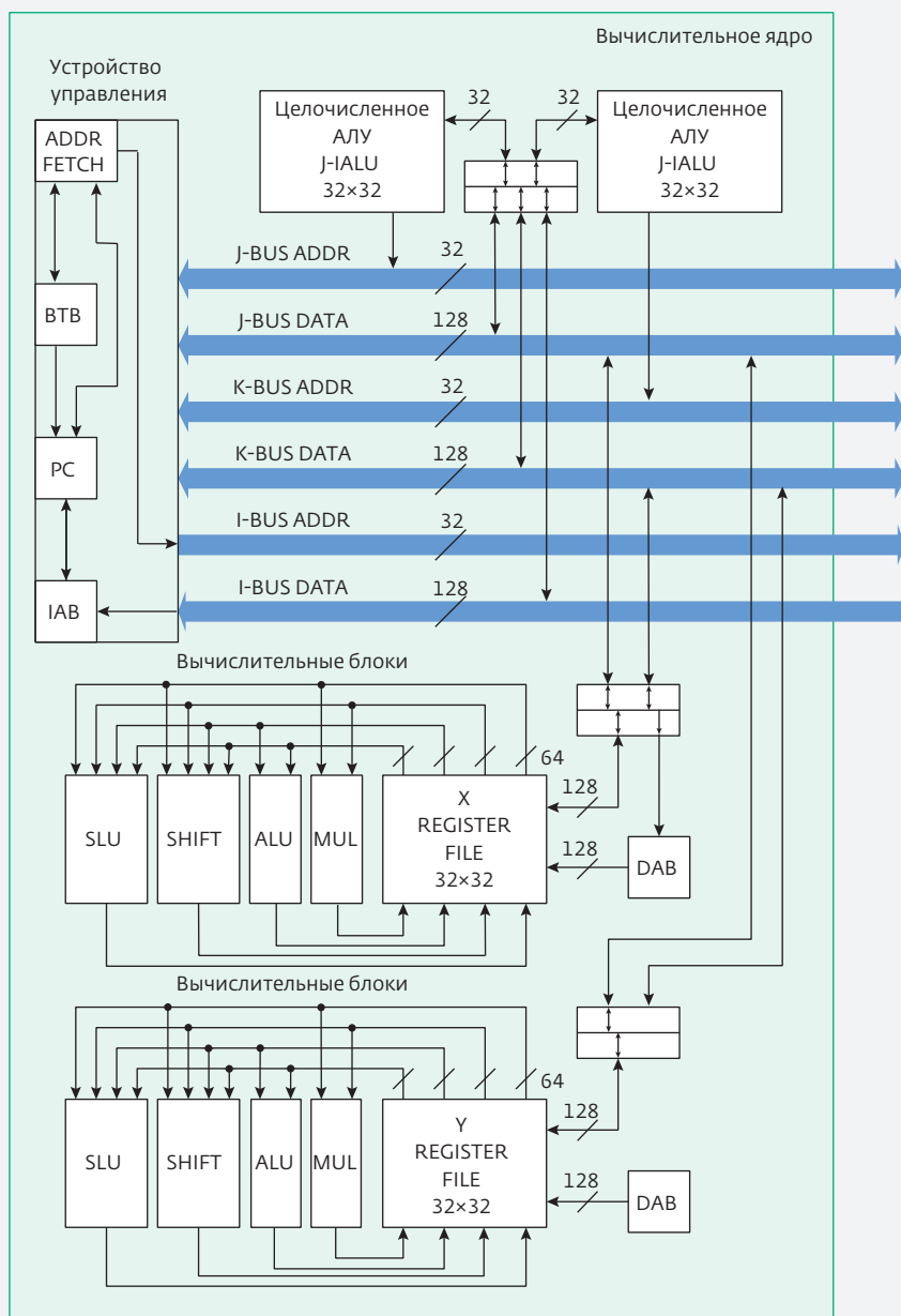
Рис.3. Структура вычислительного ядра
