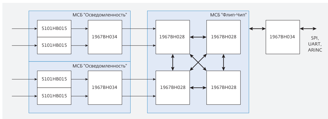
Рис.1. Структура многоканальной системы обработки данных (микросхема 5101HB015 – АЦП)
