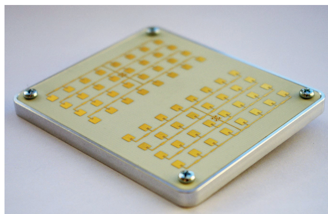
Рис. 2. Внешний вид ФАР однолучевого радара
