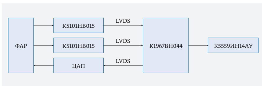
Рис. 3. Функциональная схема цифрового вычислителя однолучевого радара
