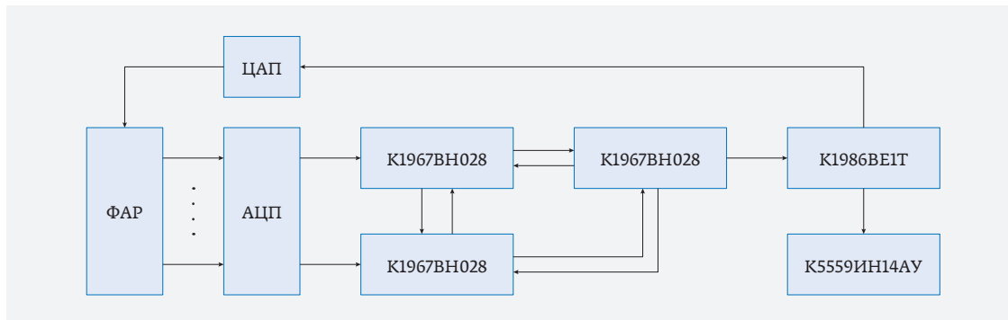
Рис. 5. Функциональная схема цифрового вычислителя многолучевого радара, работающего на частоте 24 ГГц
